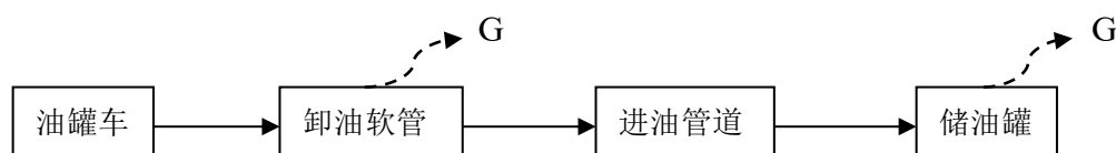
图 5-3 卸油工艺流程
