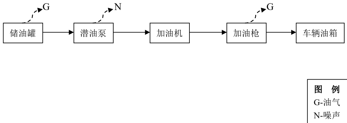
图 5-4 加油工艺流程
