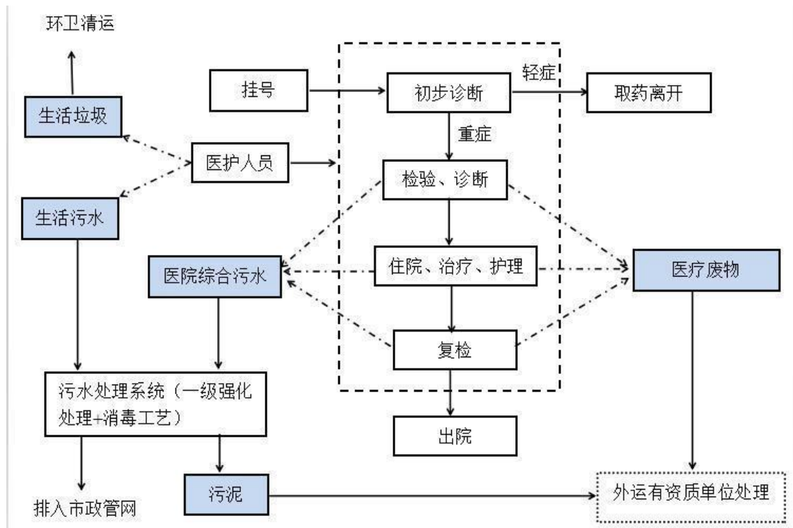
图 2-3 项目运营期产污流程图
