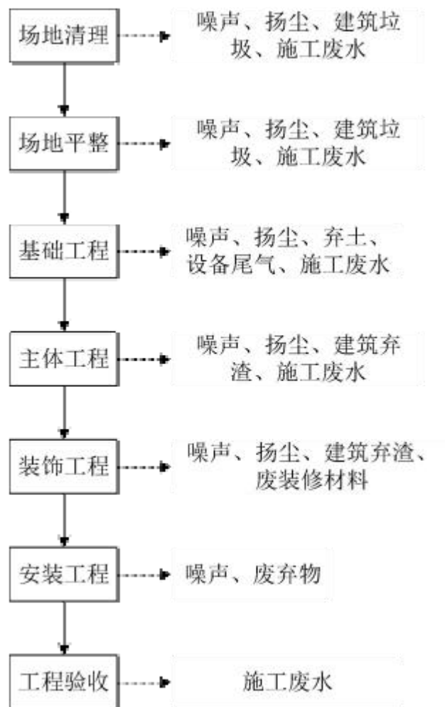
图 2-2 项目施工期工艺流程图
