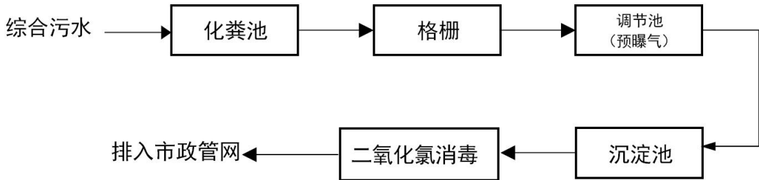
图 4-1 项目污水处理站工艺流程图
