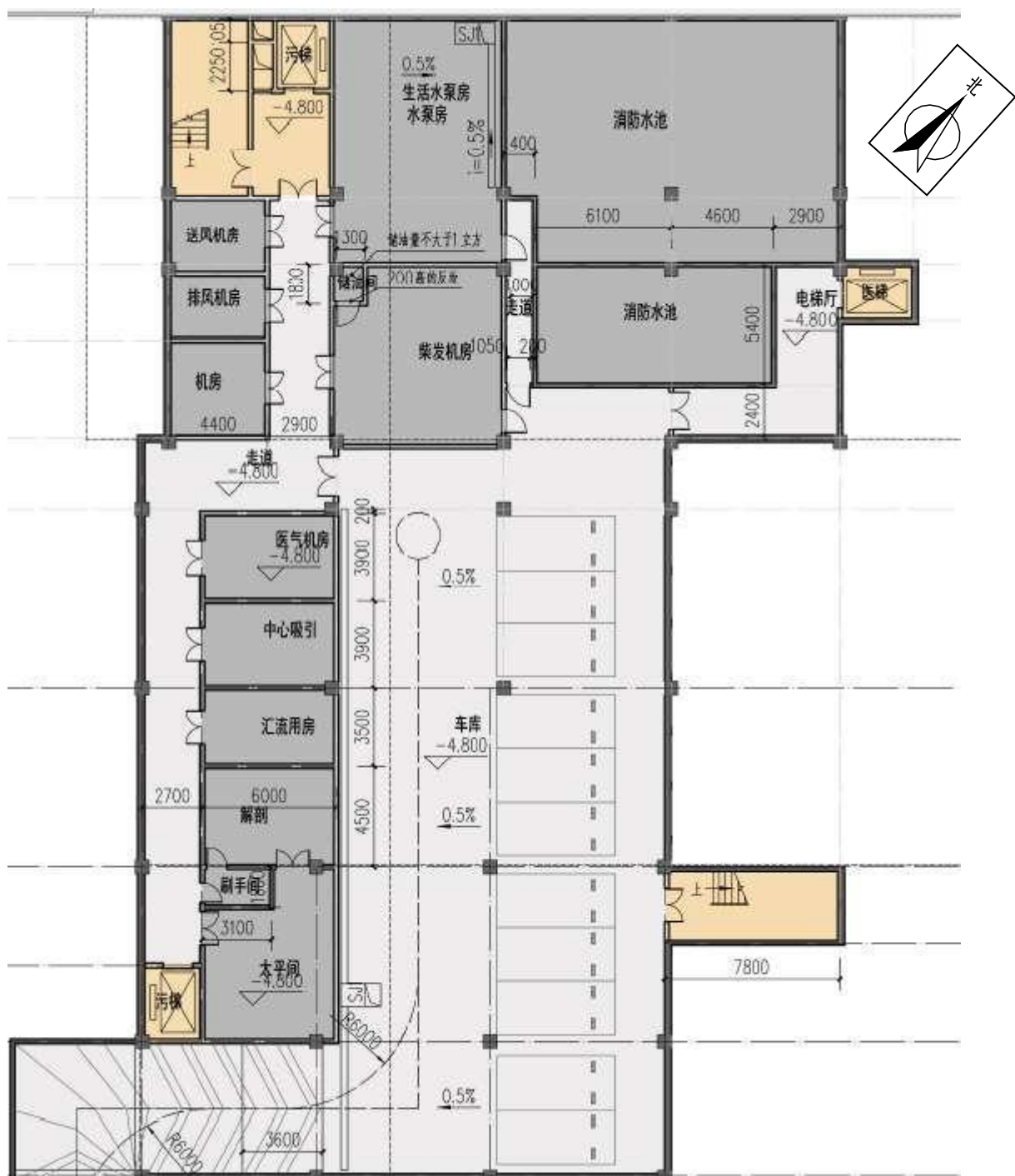
地下一层平面布置图
