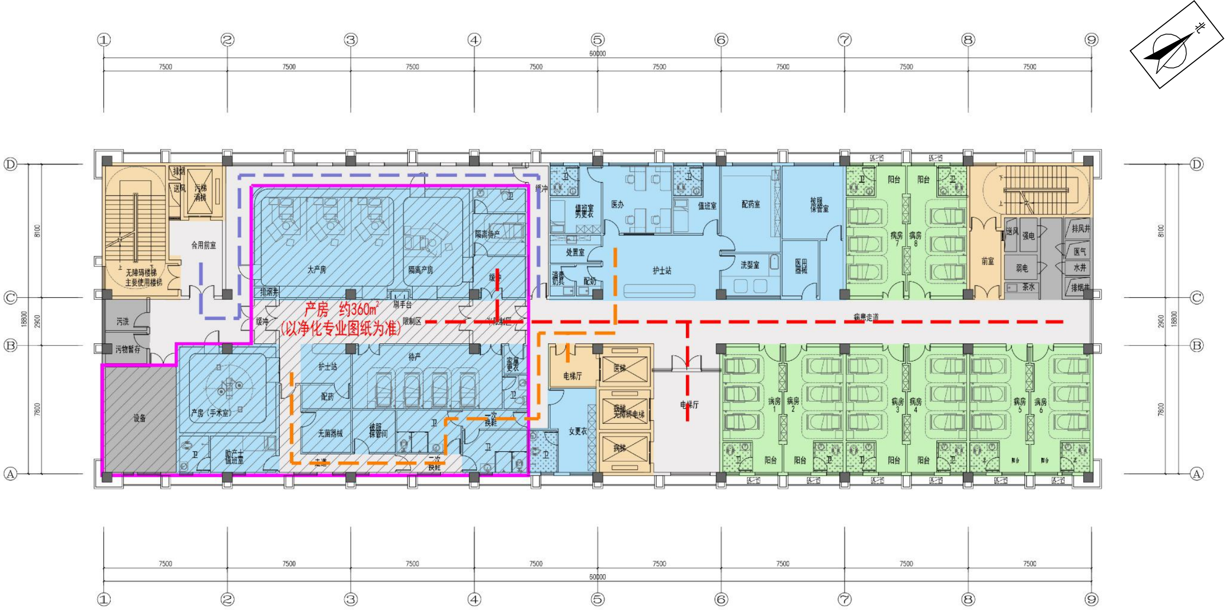
五层平面图 1:100 本层建筑面积: 1143.80m 2
