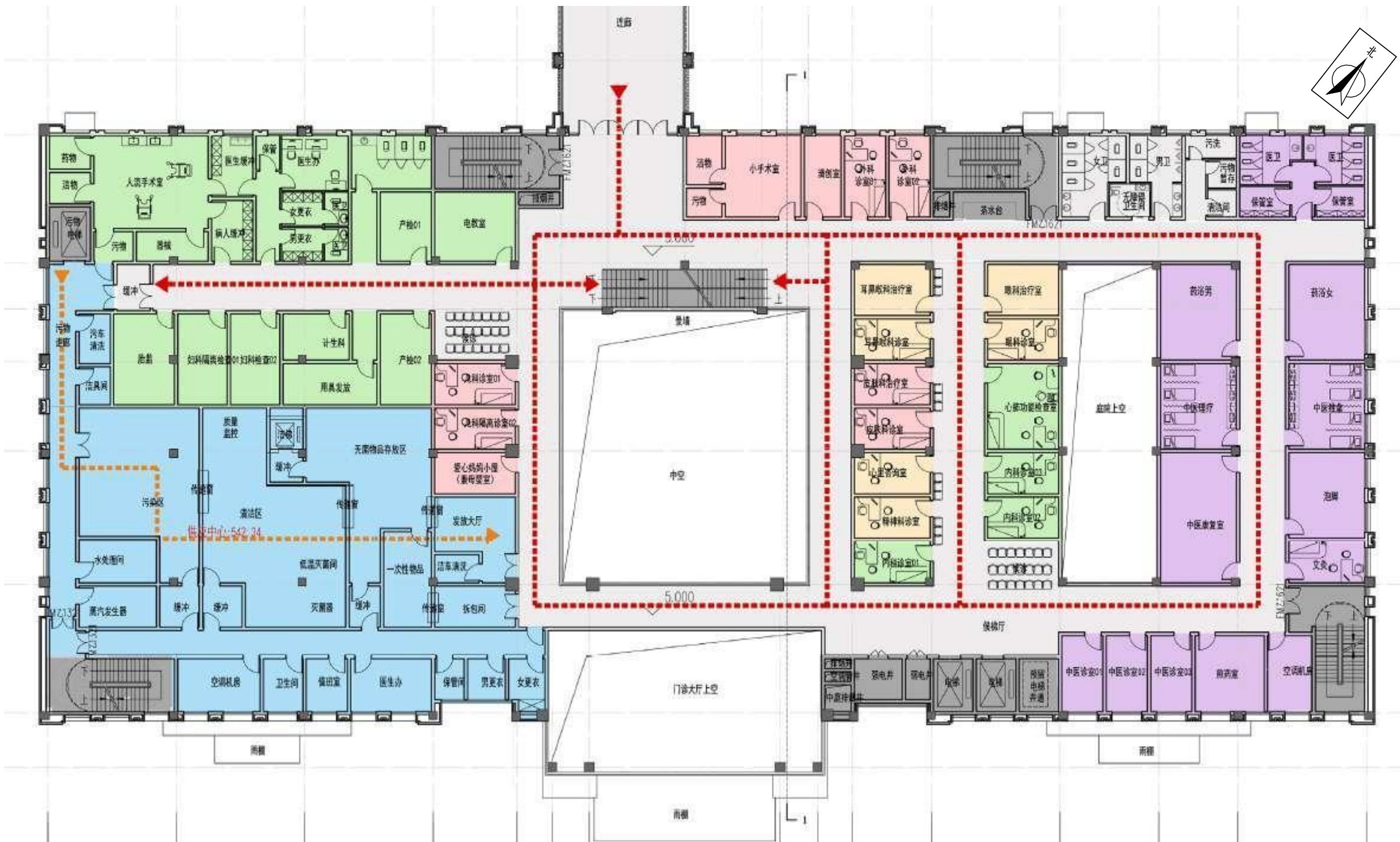
综合门诊楼二层平面布置图
