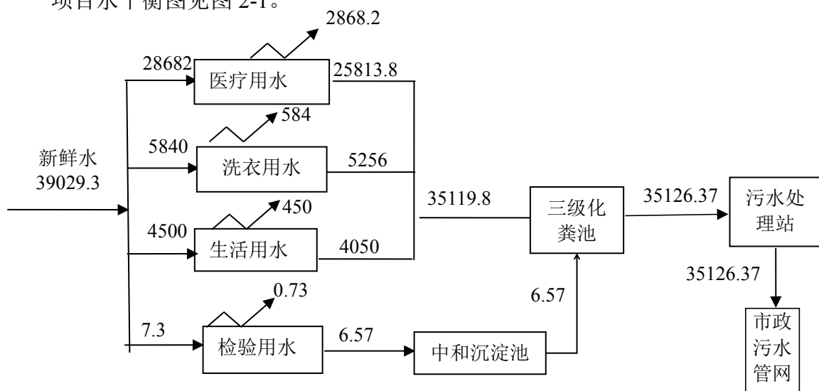
图 2-1 项目用水平衡图 单位：m 3 /a
