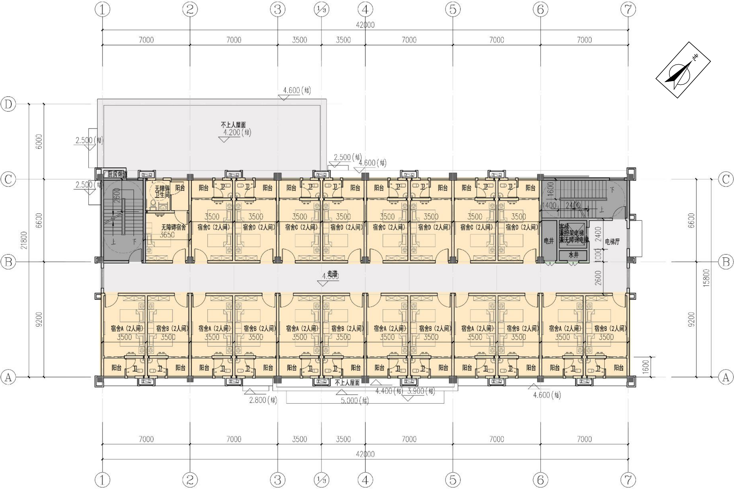
后勤楼二层、三层、四层平面布置图
