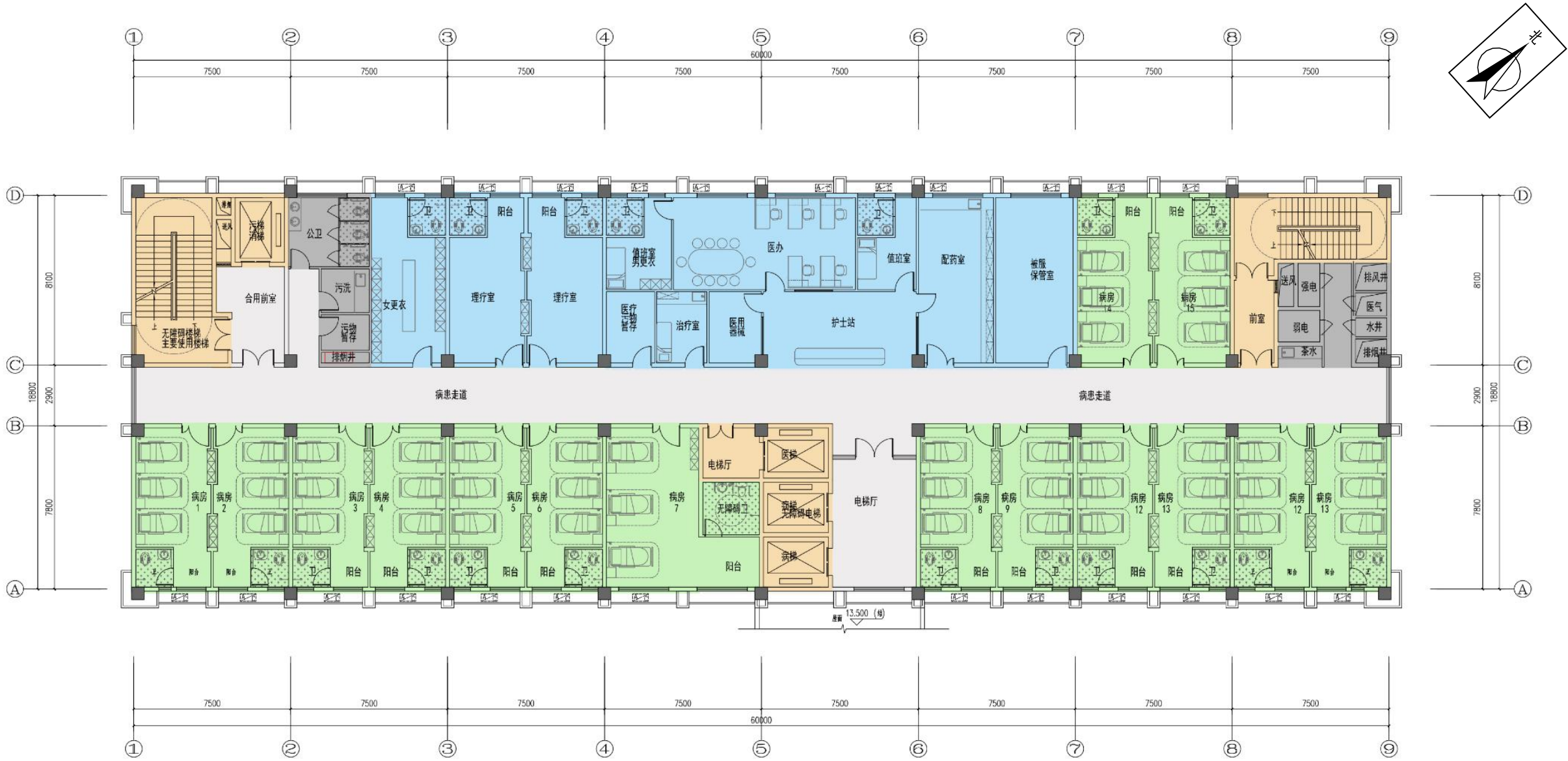
四层平面图 1:100 本层建筑面积: 1143.80m 2
