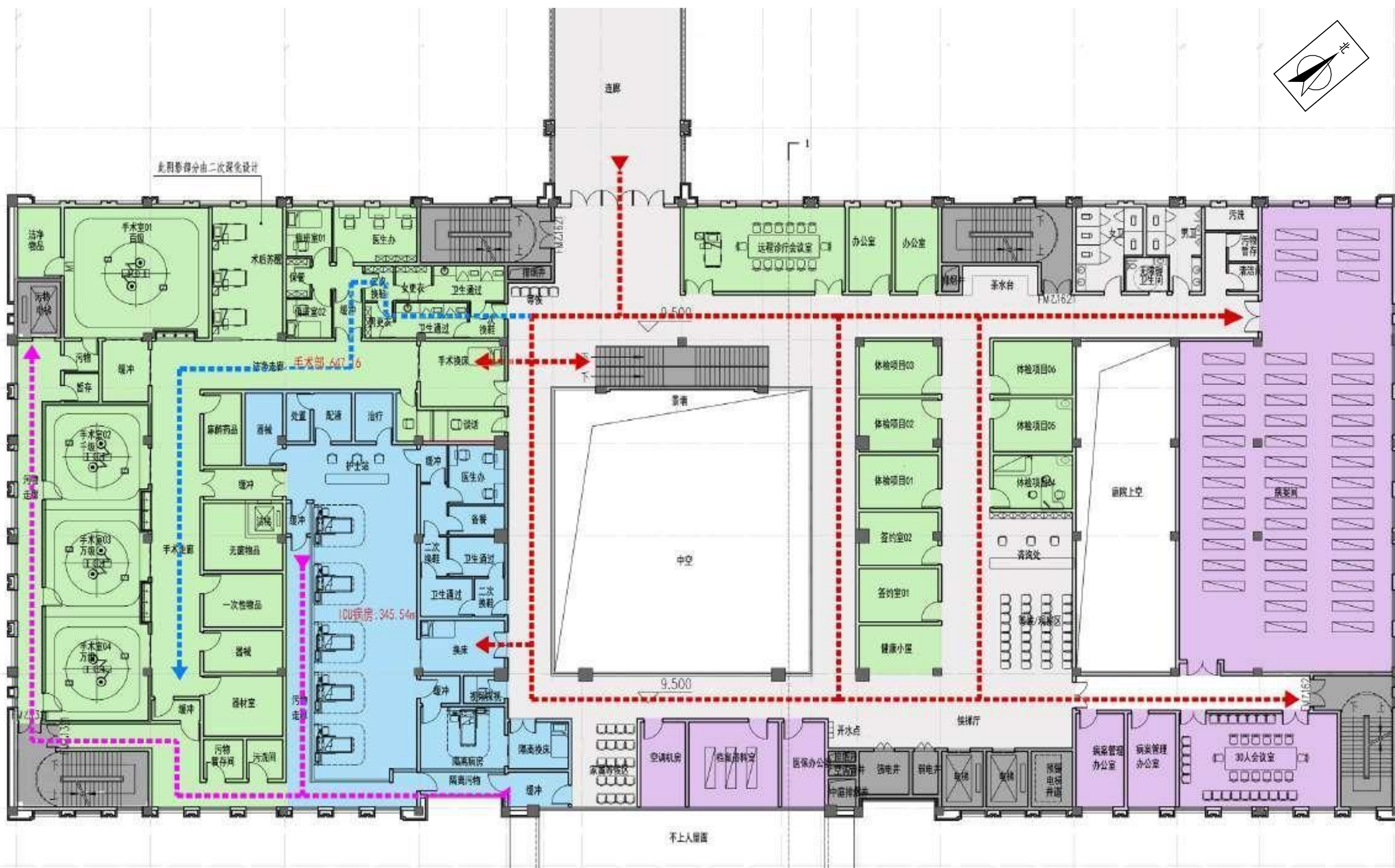
三层平面布置图
