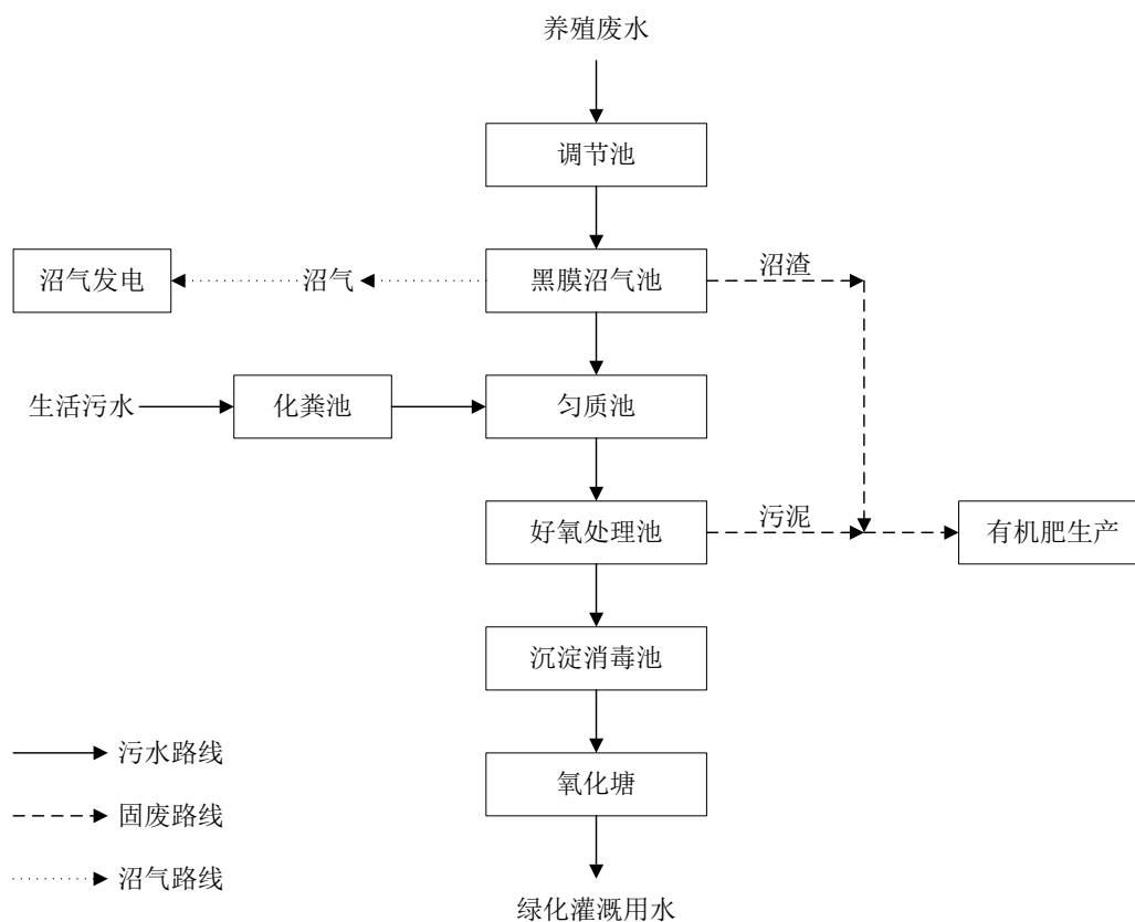
图 3.8-1 原有项目自建污水处理站工艺流程图
