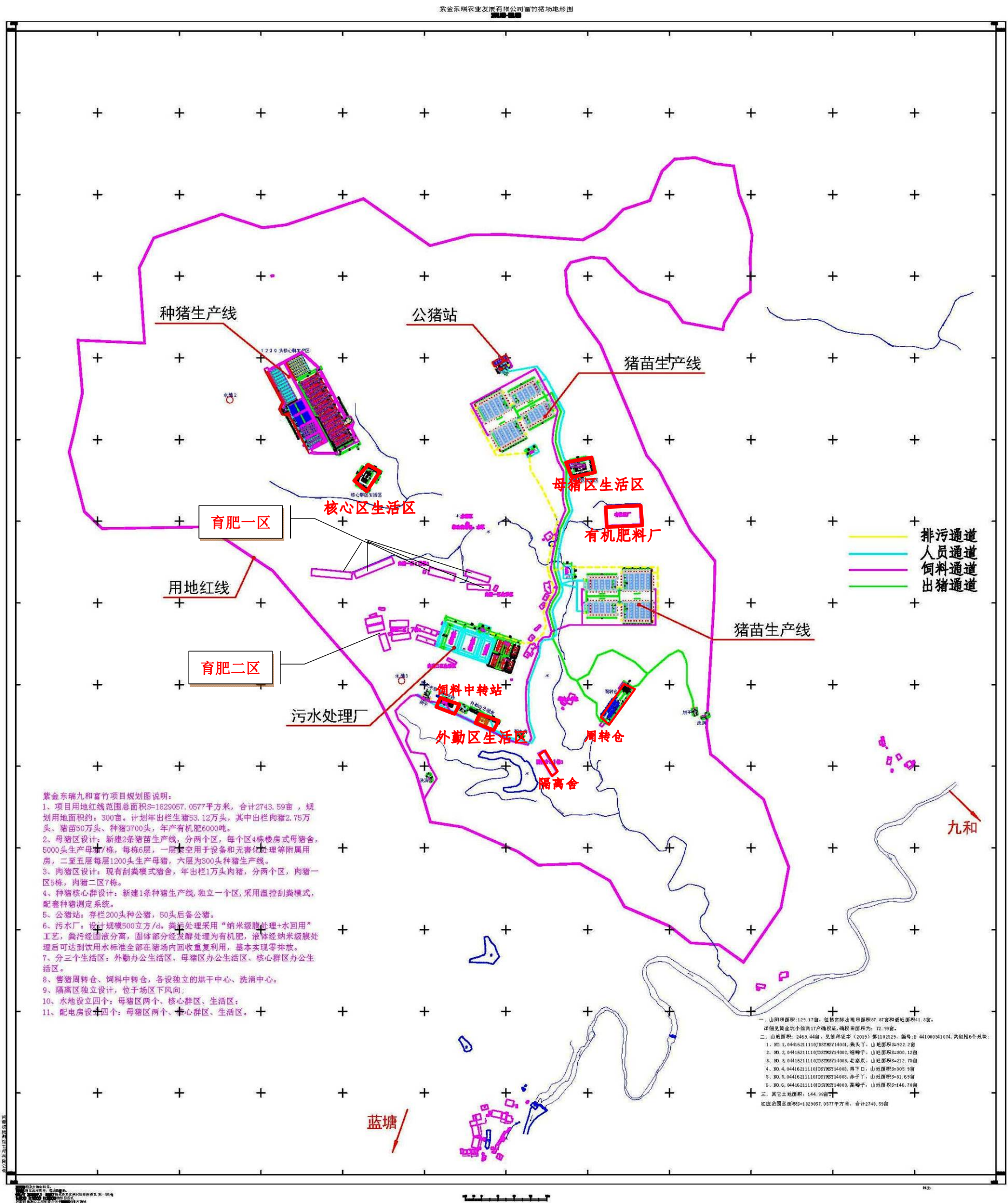
图 4.1-4 项目总平面布置图
