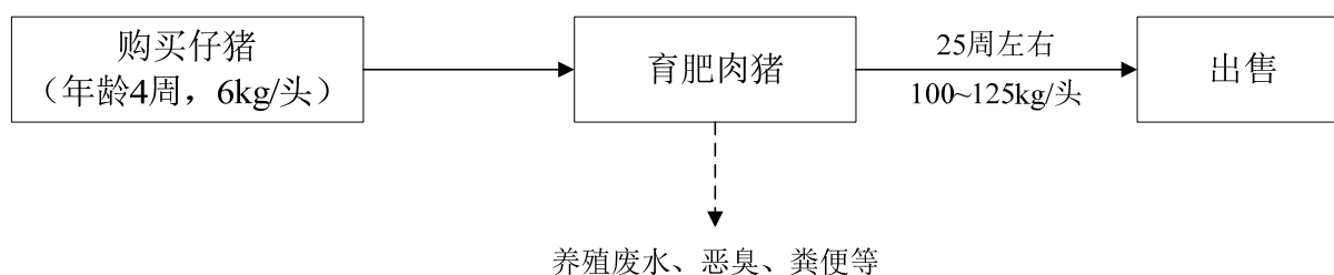
图 3.6-1 原有项目养猪生产工艺流程图
