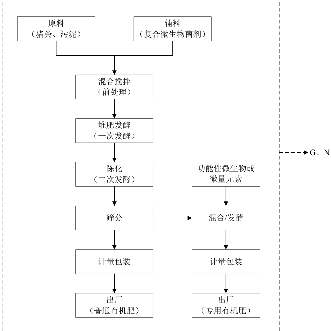
图 3.6-3 有机肥料生产工艺流程图
