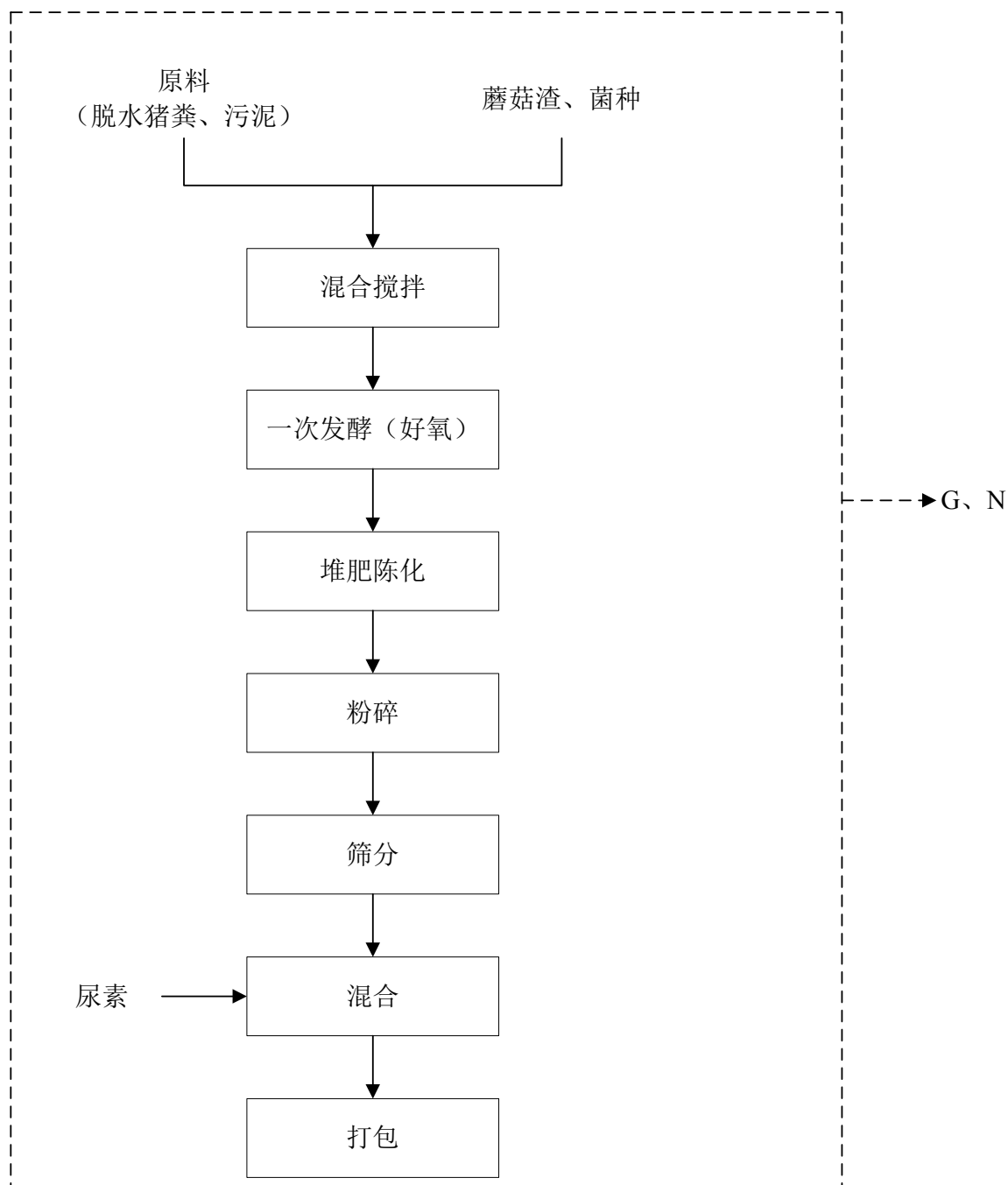
图 4.4-4 有机肥料生产工艺流程图
