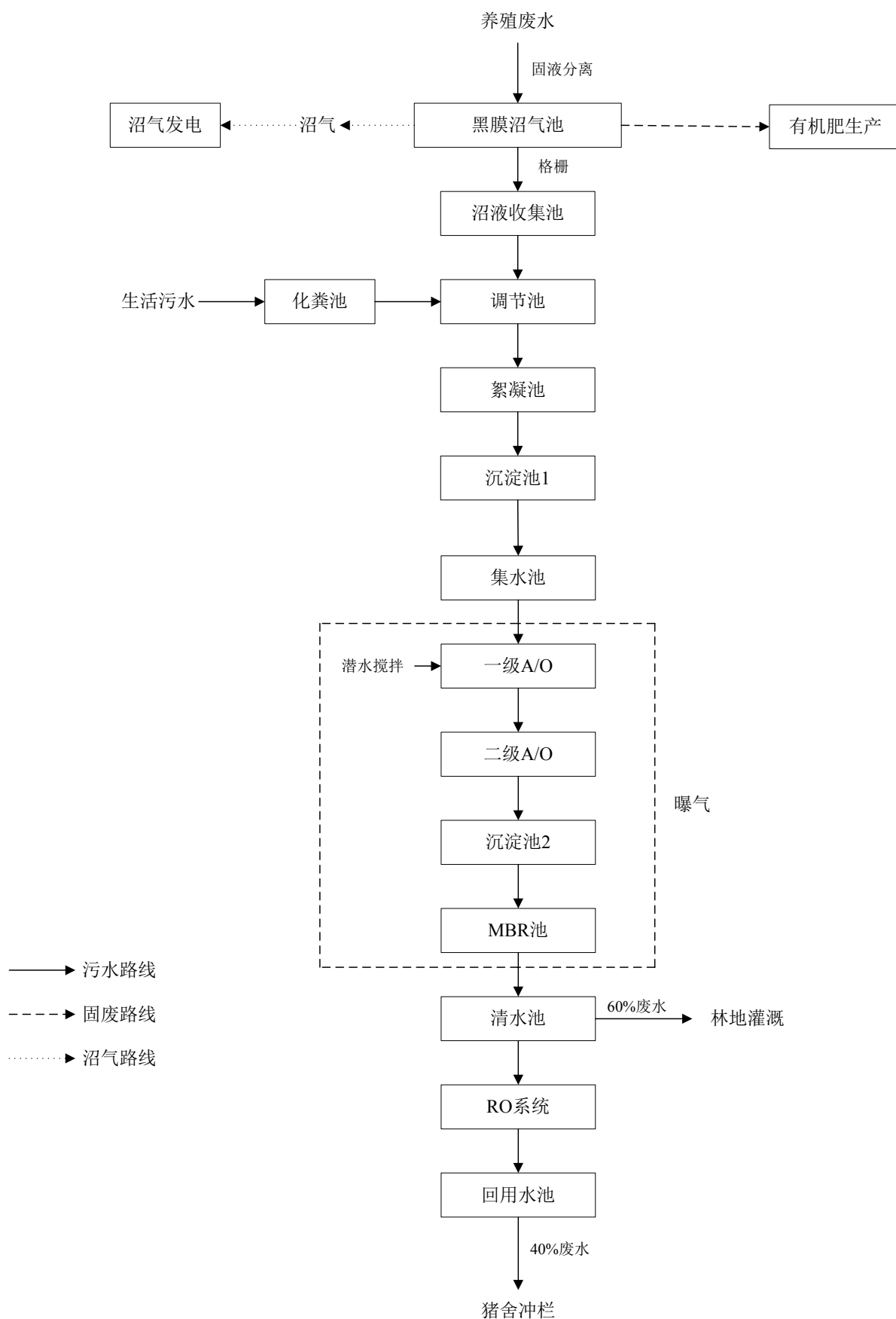
图 8.2-1 项目污水处理站工艺流程图
