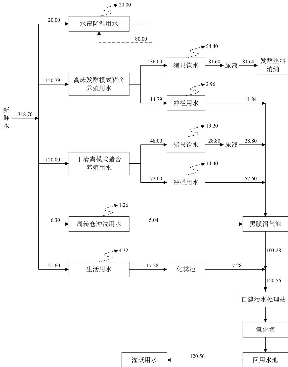
图 3.7-1 原有项目水平衡图
