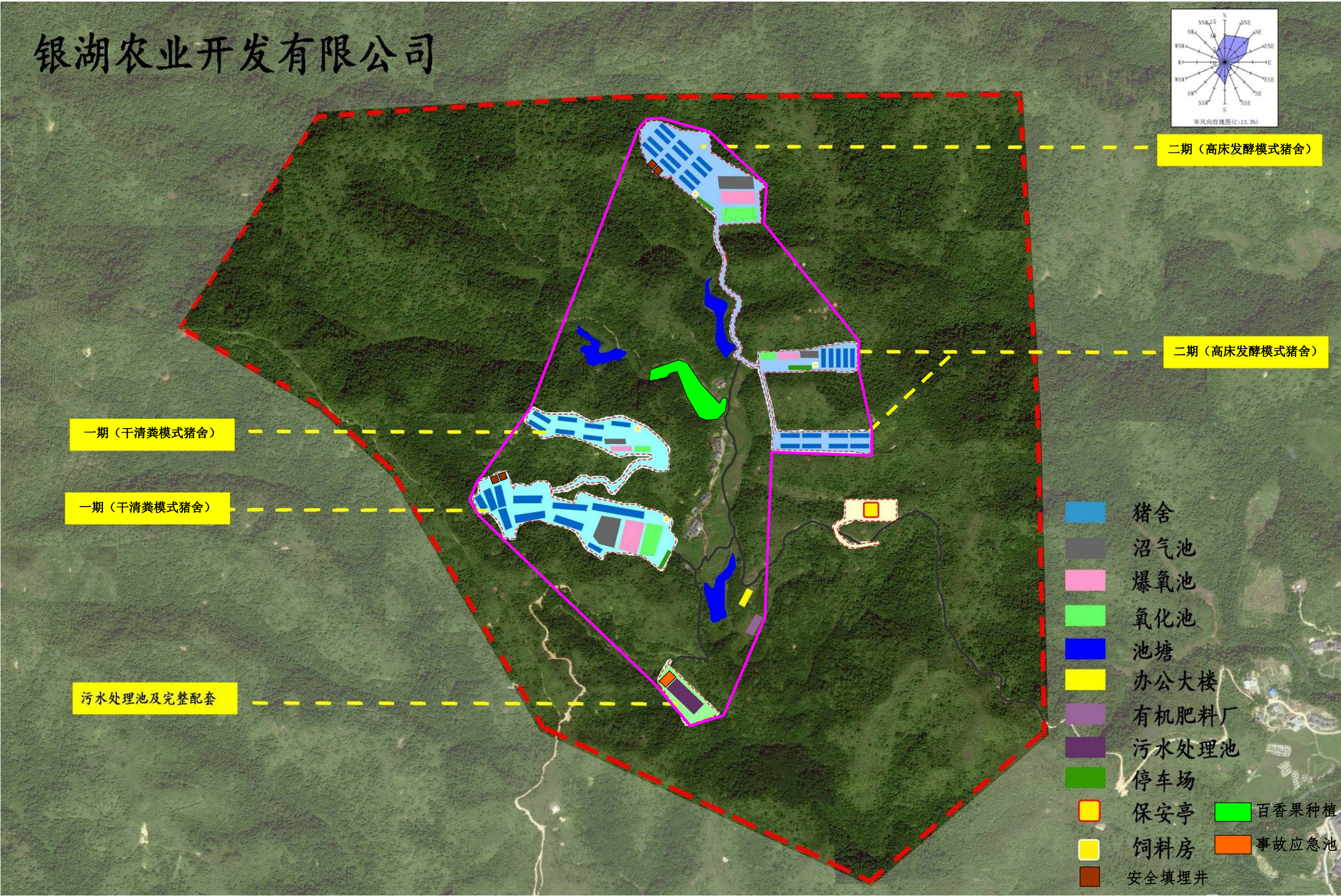
图 3.2-1 原有项目总平面布置图
