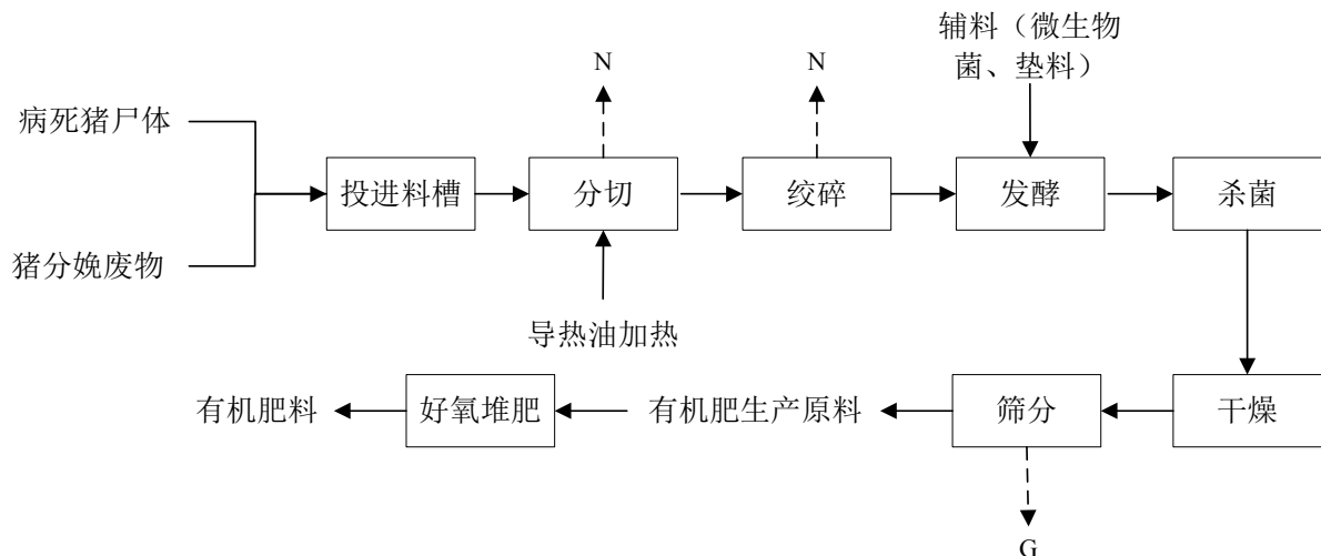
图 4.4-6 病死猪尸体及分娩废物无害化处理工艺流程图
