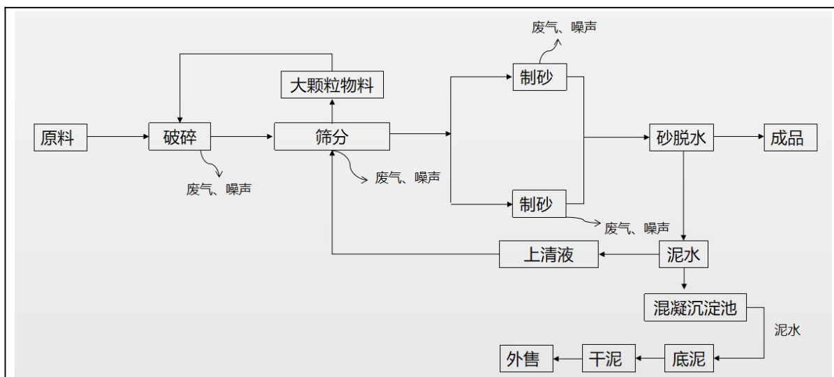
图5-2 营运期砂石生产工艺流程及产污节点
