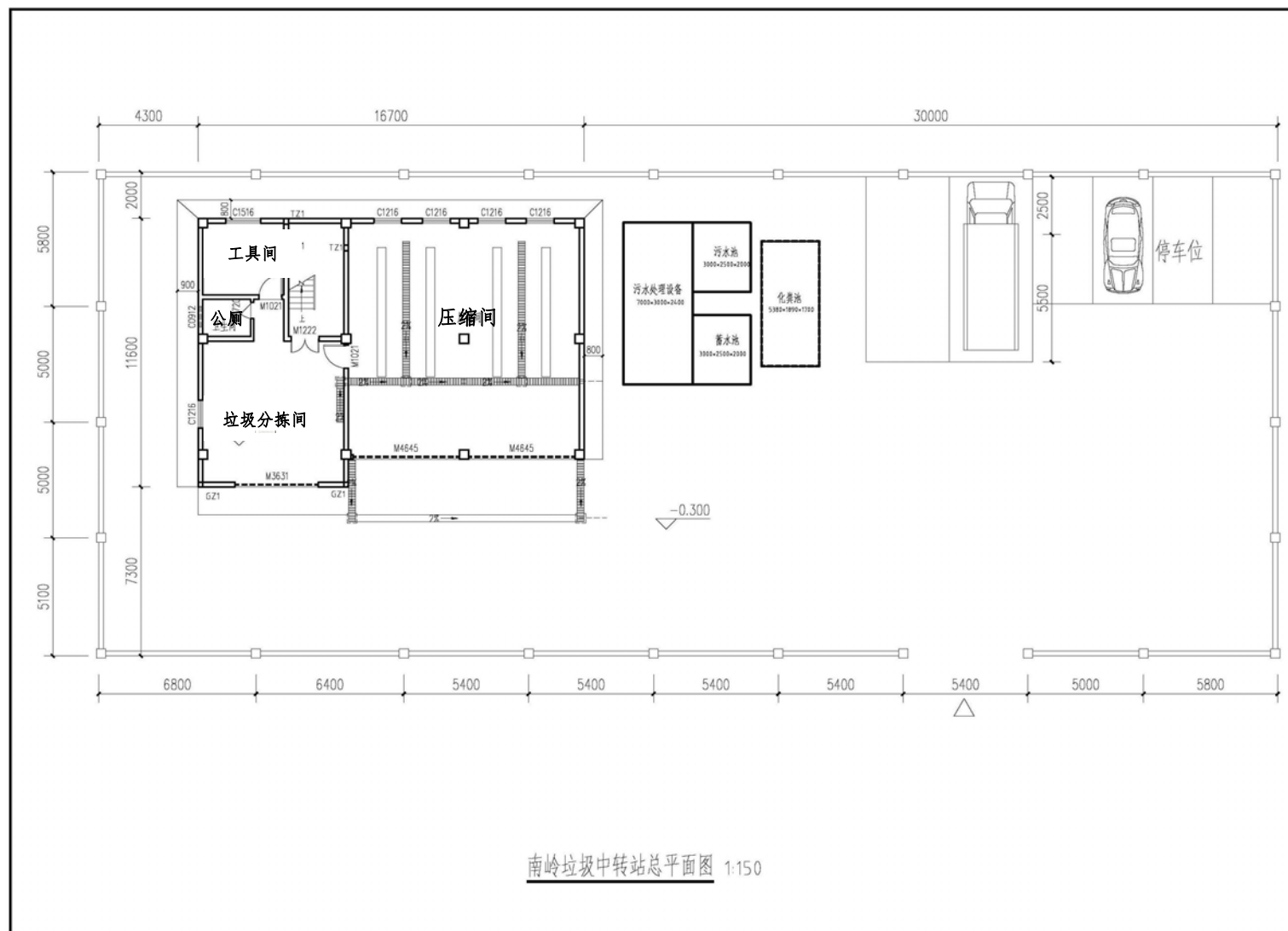
附图七 项目总平面布置图
