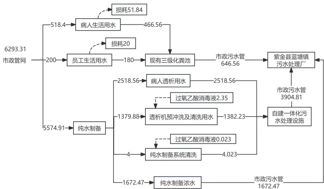
图 2-1 项目用水平衡图 单位: \text{m}^3/\text{a}
