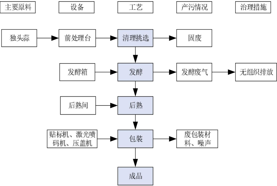
图2-5 黑蒜生产工艺流程及产污环节图
