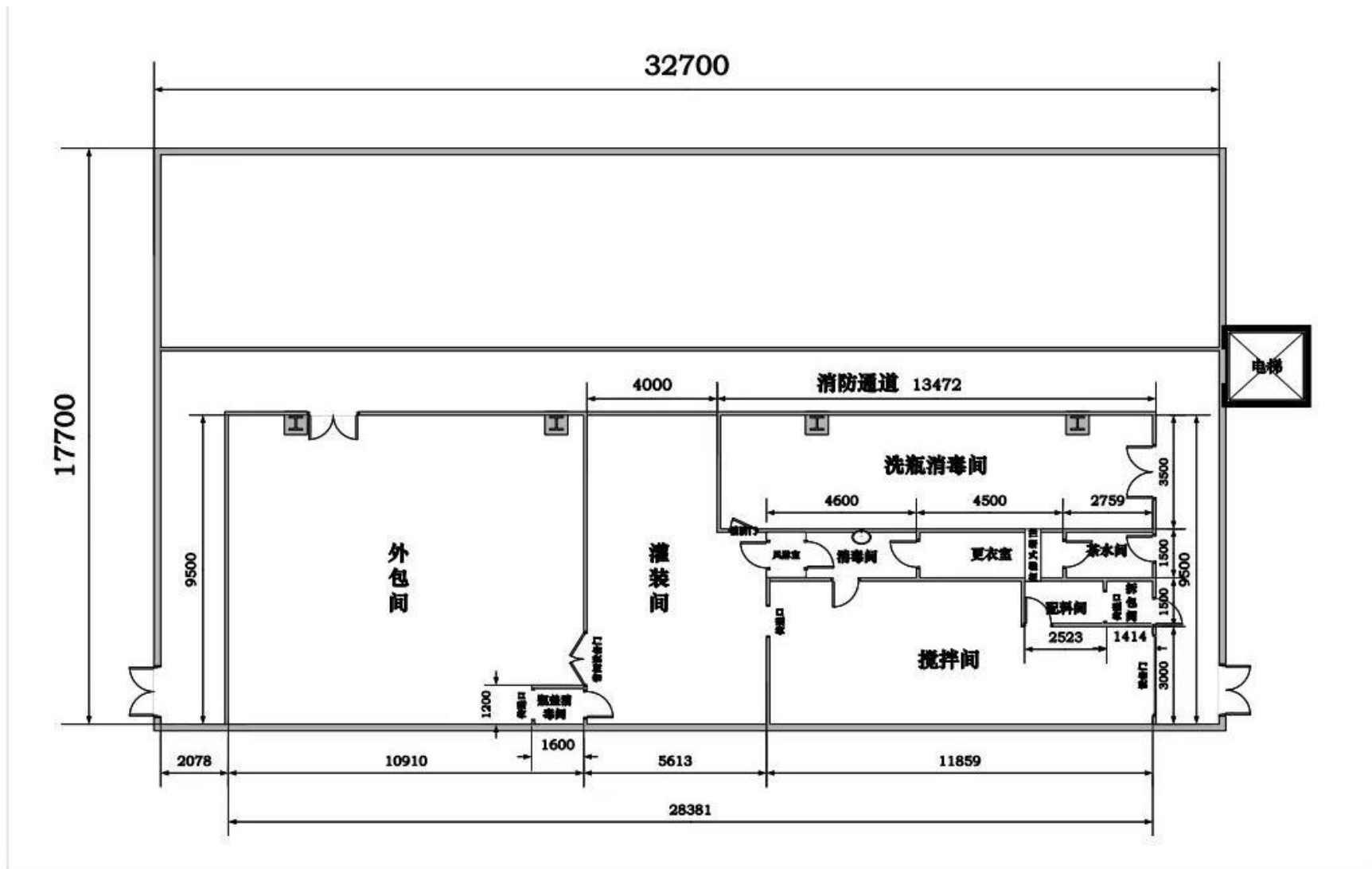
附图4.1、2#厂房1楼平面布置图
