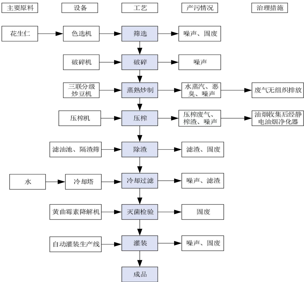
图2-4 花生油生产工艺流程及产污环节图
