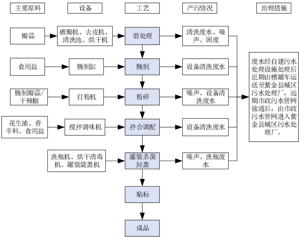
图2-3 椒酱工艺流程及产污环节图
