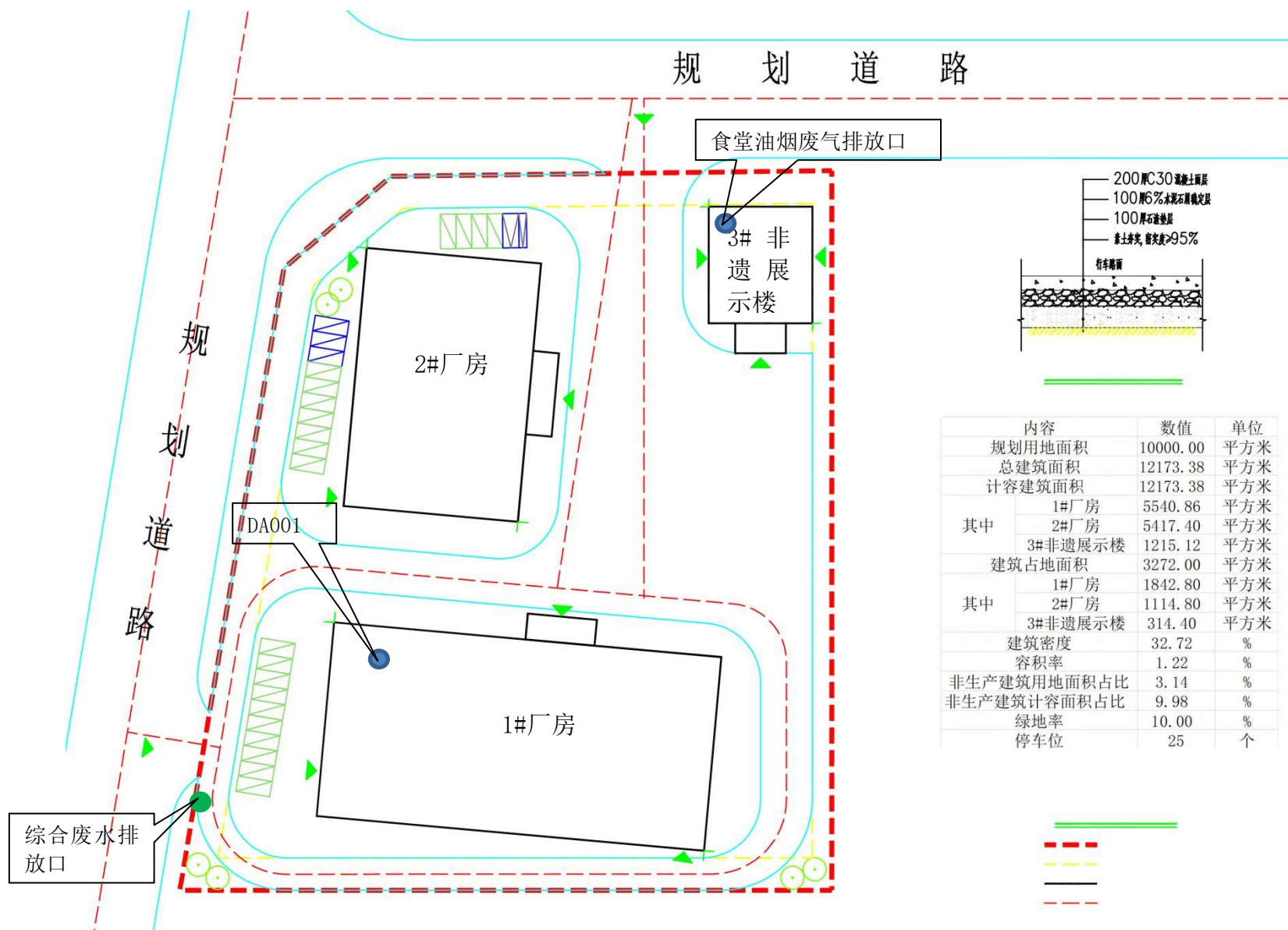
附图4、平面布置图
