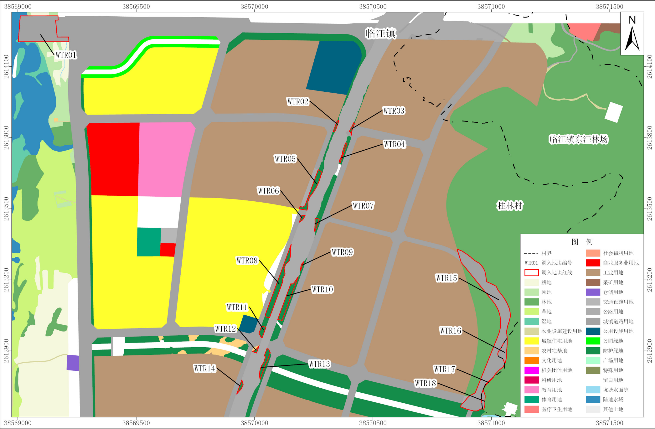
河源市紫金县城镇建设用地规模调入地块土地使用规划局部图（WTR01—WTR18）（落实后）
