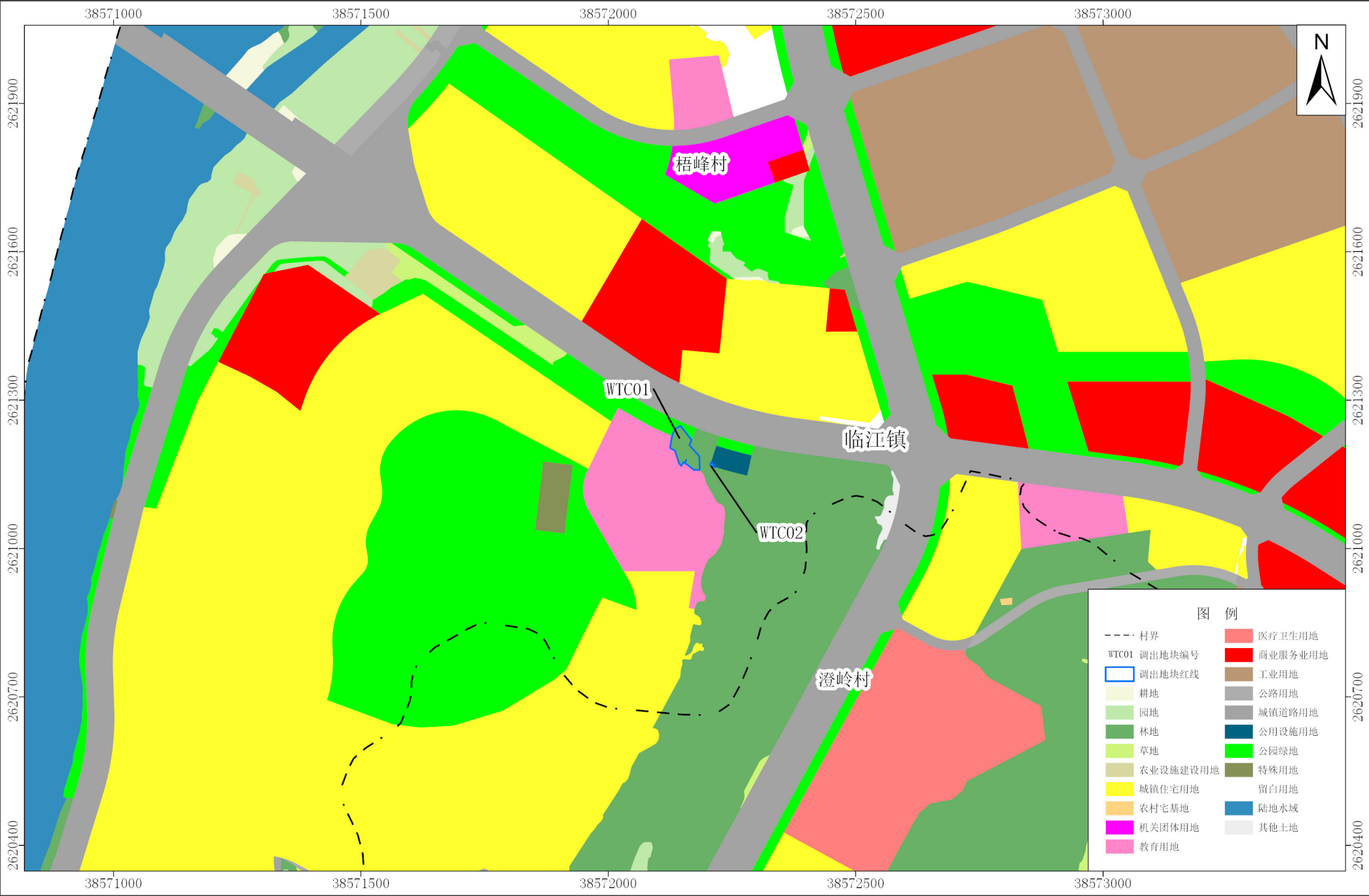
河源市紫金县城镇建设用地规模调出地块土地使用规划局部图（WTC01—WTC02）（落实后）
